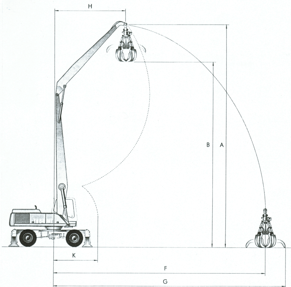
Knickarm D 84.16i - Nutzlänge 6900 mm Ausrüstung: A 84.32, C 84.5i, D 84.16i, E 850
